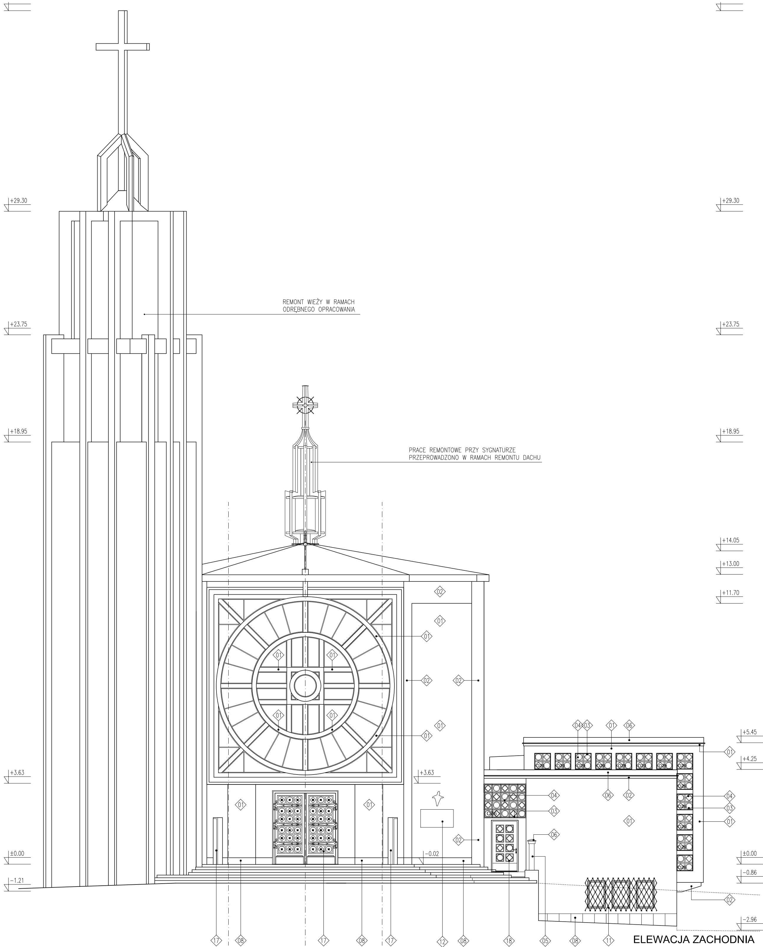
ELEWACJA ZACHODNIA
