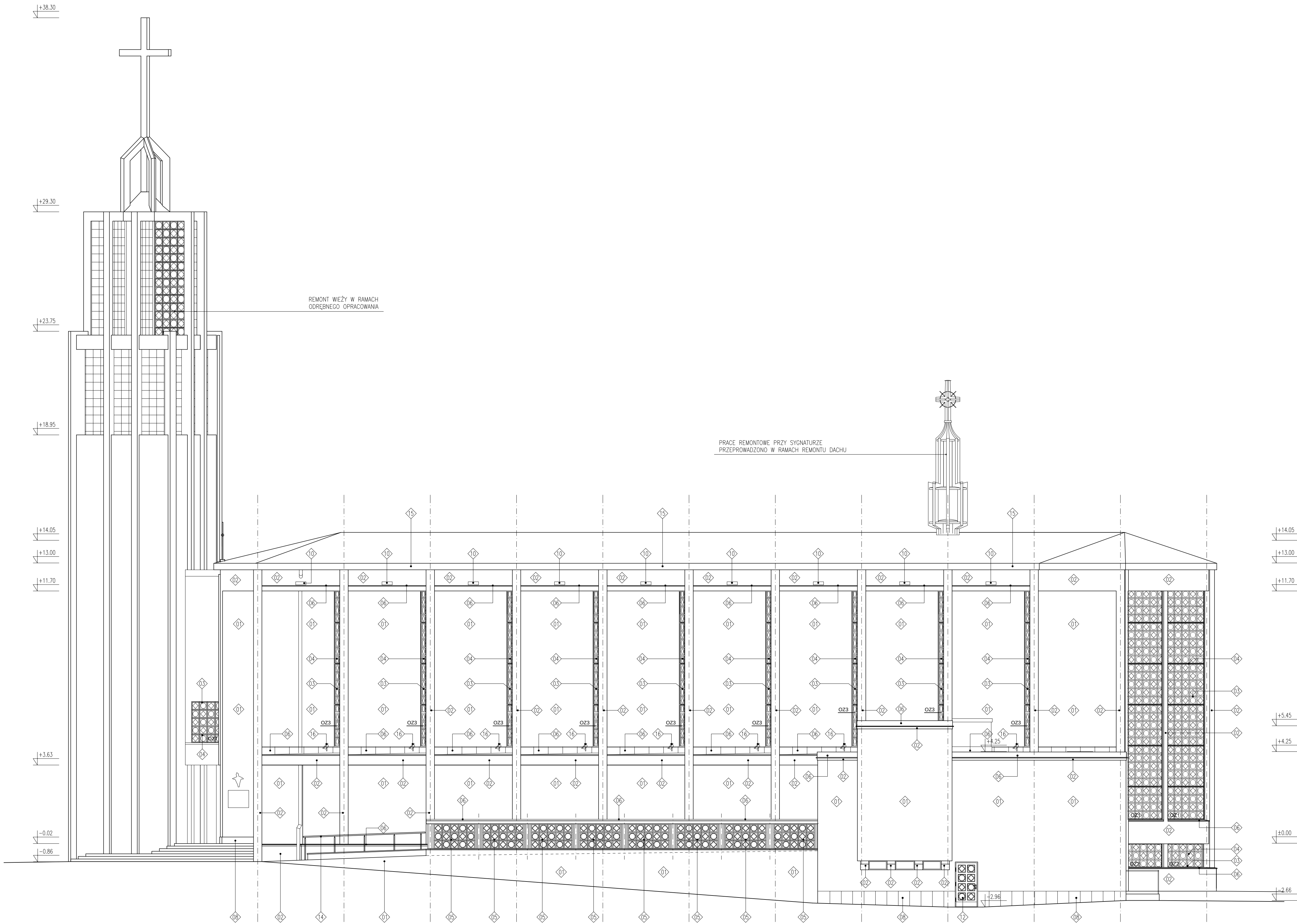
ELEWACJA POŁUDNIOWA
