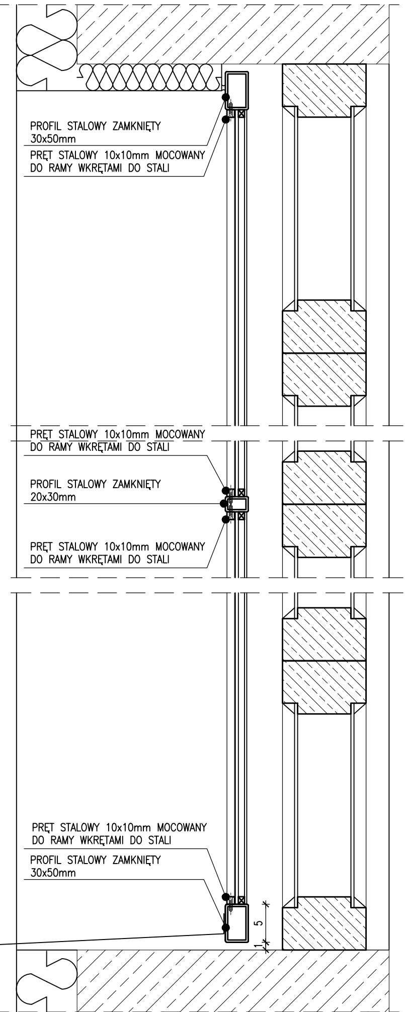
PRZEKRÓJ
