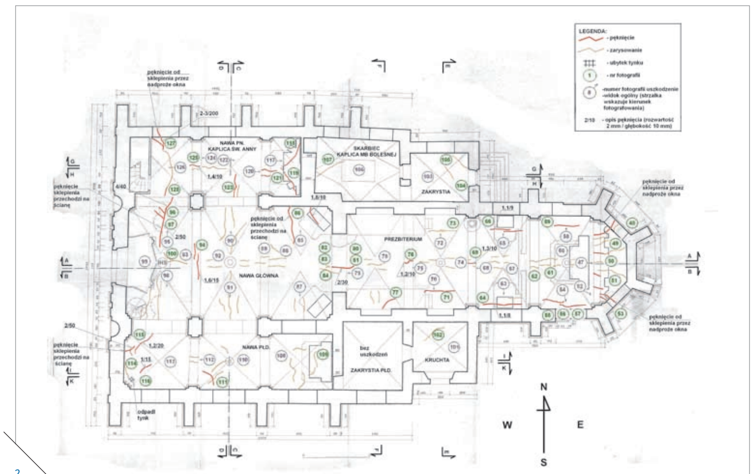
2. Kościół św. Mikołaja w Krakowie. Inwentaryzacja uszkodzeń sklepienia.
