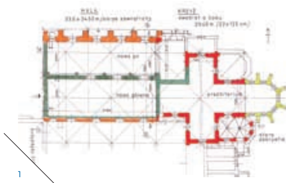
1. Rzut kościoła, rozwarstwienie gotyckich faz budowy: kolor ciemnoczerwony – ok. poł. XIII w.; kolor jasnoczerwony – trzecia ćw. XIII w.; kolor jasnozielony – lata 1400-1436; kolor ciemnozielony – po 1465 r.
